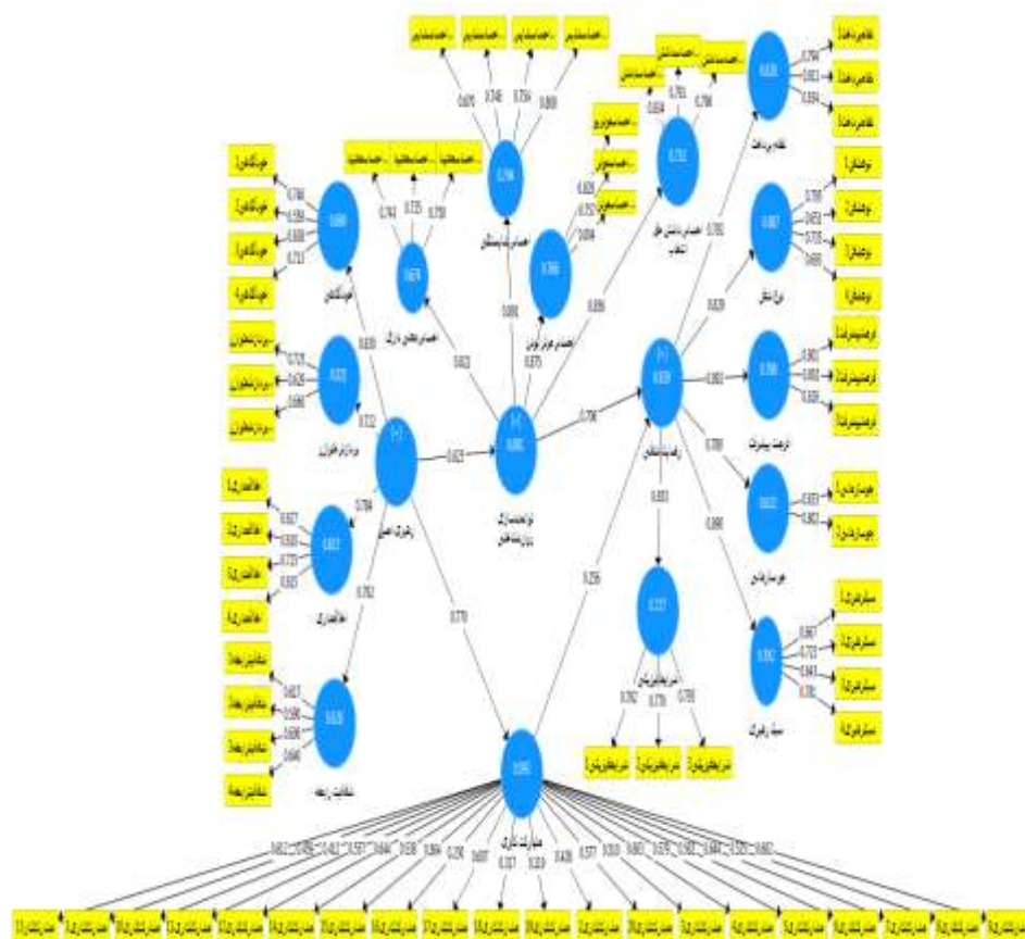
شکل ۲: مدل در حالت ضرایب مسیر R^2
